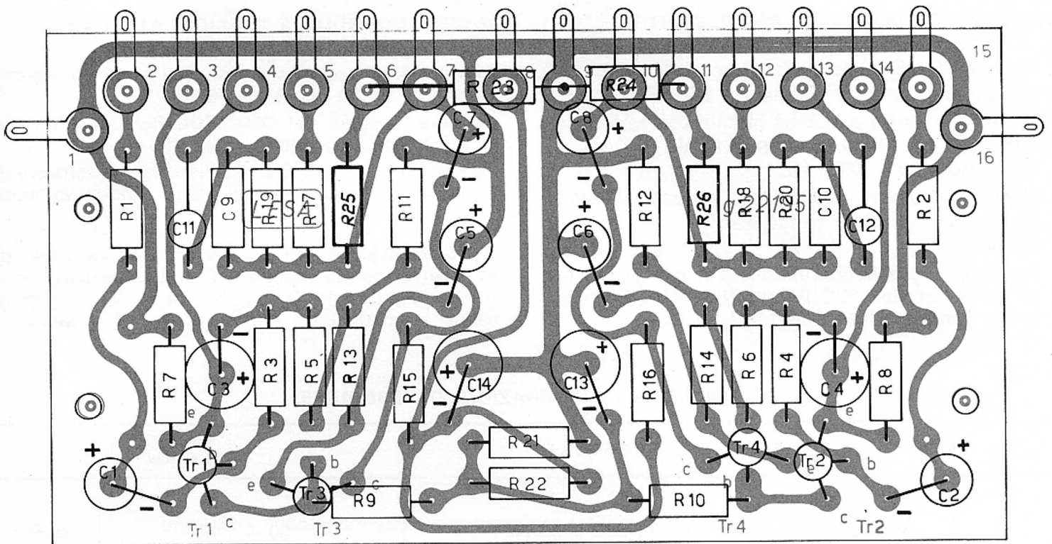
Circuito stampato stadio preamplificatore equalizzatore.
