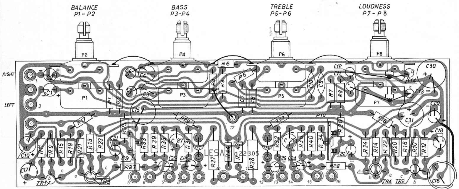
Circuito stampato stadio amplificatore (esclusi stadi finali).
